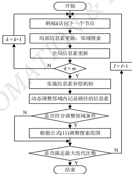
图 3 算法流程图
